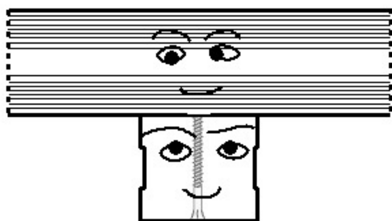
角スタッド+直交角スタッド “カクスタスクリュー串刺し工法”
